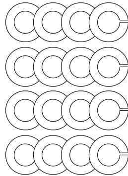
Z14 Ø12.2xØ21.5x3.0T
