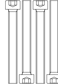
Z23 M10x1.5Px85L
