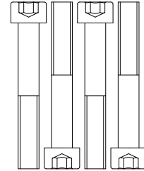
Z11 M10x1.5Px70L-35L
