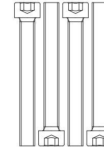
Z23 M10x1.5Px85L
