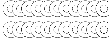
Z13 Φ10.2xΦ22x2.0T
