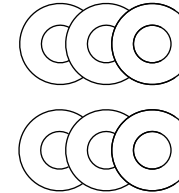
Z13 Ø10.2xØ22x2.0T
