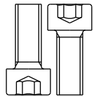
Z20 M10x1.5Px25L
