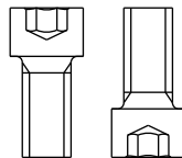
Z03 M12x25L
