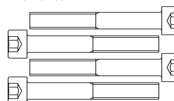
Z12 M10x70L-35L
