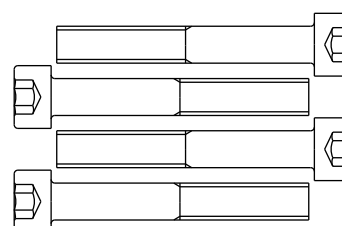
Z12 M10x70L-35L
