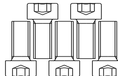
Z08 M10x25L
