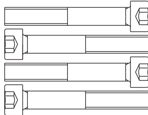
Z05 M10x1.5Px70L-35L
