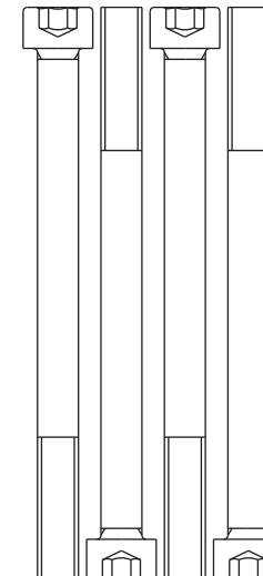
Z15 M10x1.5Px130L-35L
