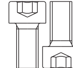
Z15 M10x1.5Px130L-35L
