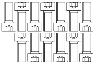
Z04 M10x1.5Px25L
