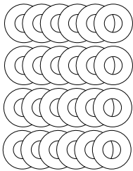
Z10 Φ10.2xΦ22.0x2.0T
