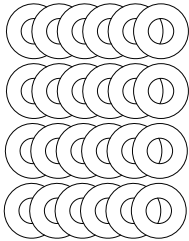
Z10 Φ10.2xΦ22.0x2.0T
