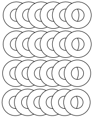
Z10 Φ10.2xΦ22.0x2.0T
