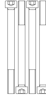
Z08 M10x1.5Px125L-35L
