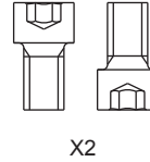
Z04 M12x20L
