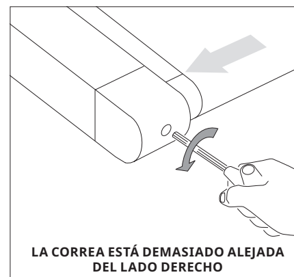
APRIETE DEL LADO DERECHO DEL RODILLO
