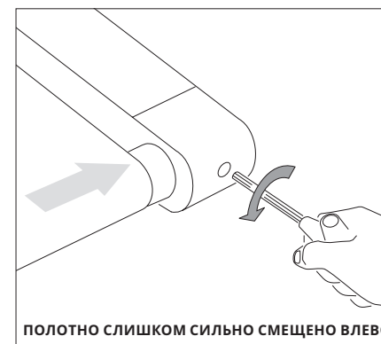
ПОЛОТНО СЛИШКОМ СИЛЬНО СМЕЩЕНО ВПРАВО
